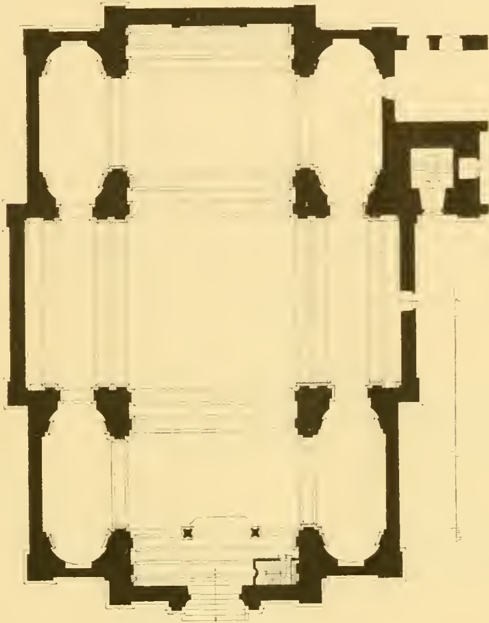
Fig. 68. Konviktskirche zu Ehingen. Grundriß.
